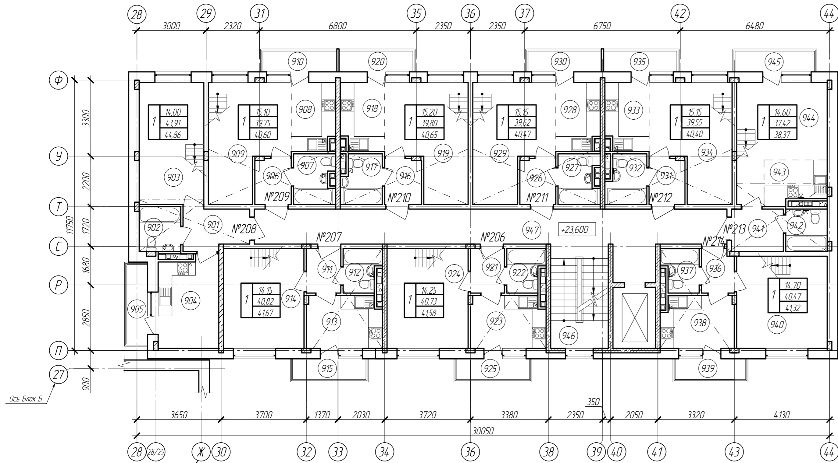
Компоновочная схема многоквартирного дома
