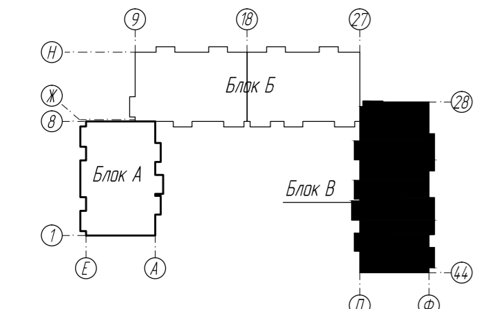
Компоновочная схема многоквартирного дома
